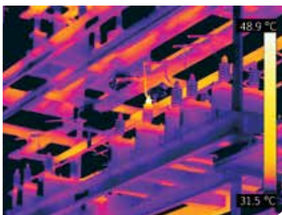
Bobina de transformador defectuosa frente al cielo frío
